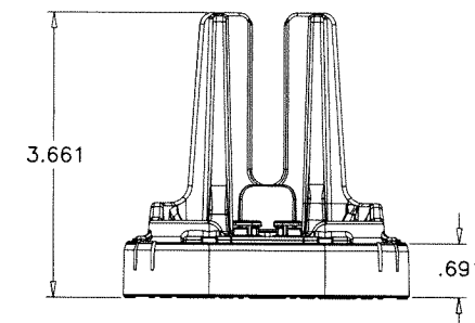
INSTAFLASH 2 MOUNT CAST ALUMINUM (Fy MIN. = 23 KSI) (Fu MIN. = 47 KSI)
